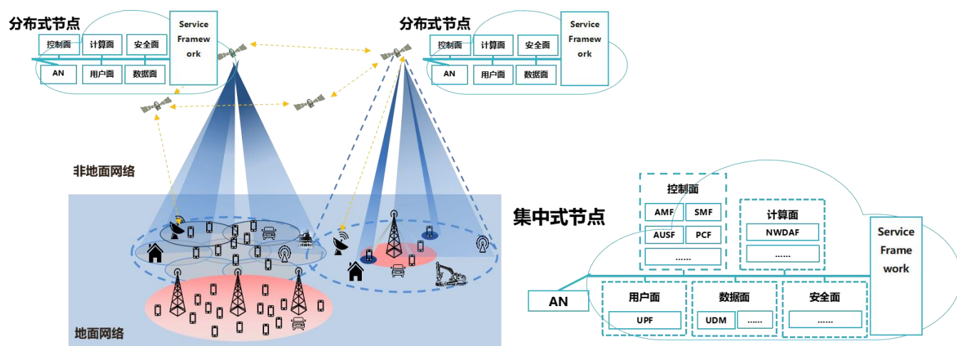
图 1 天地一体分布式自治网络结构参考
