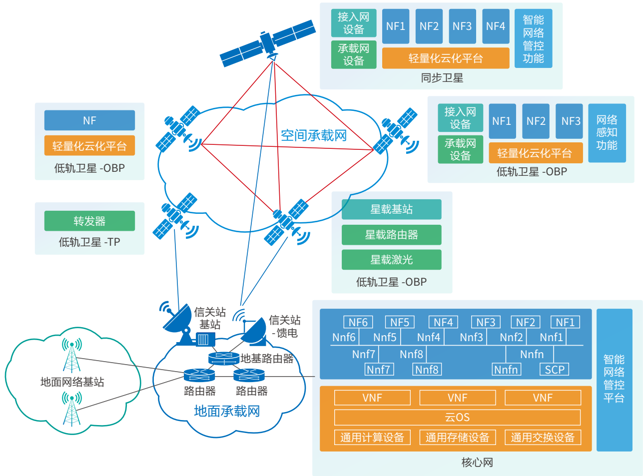
图2-星地融合通信网络架构
