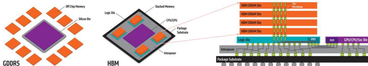
图表26： GDDR 与 HBM 差异
